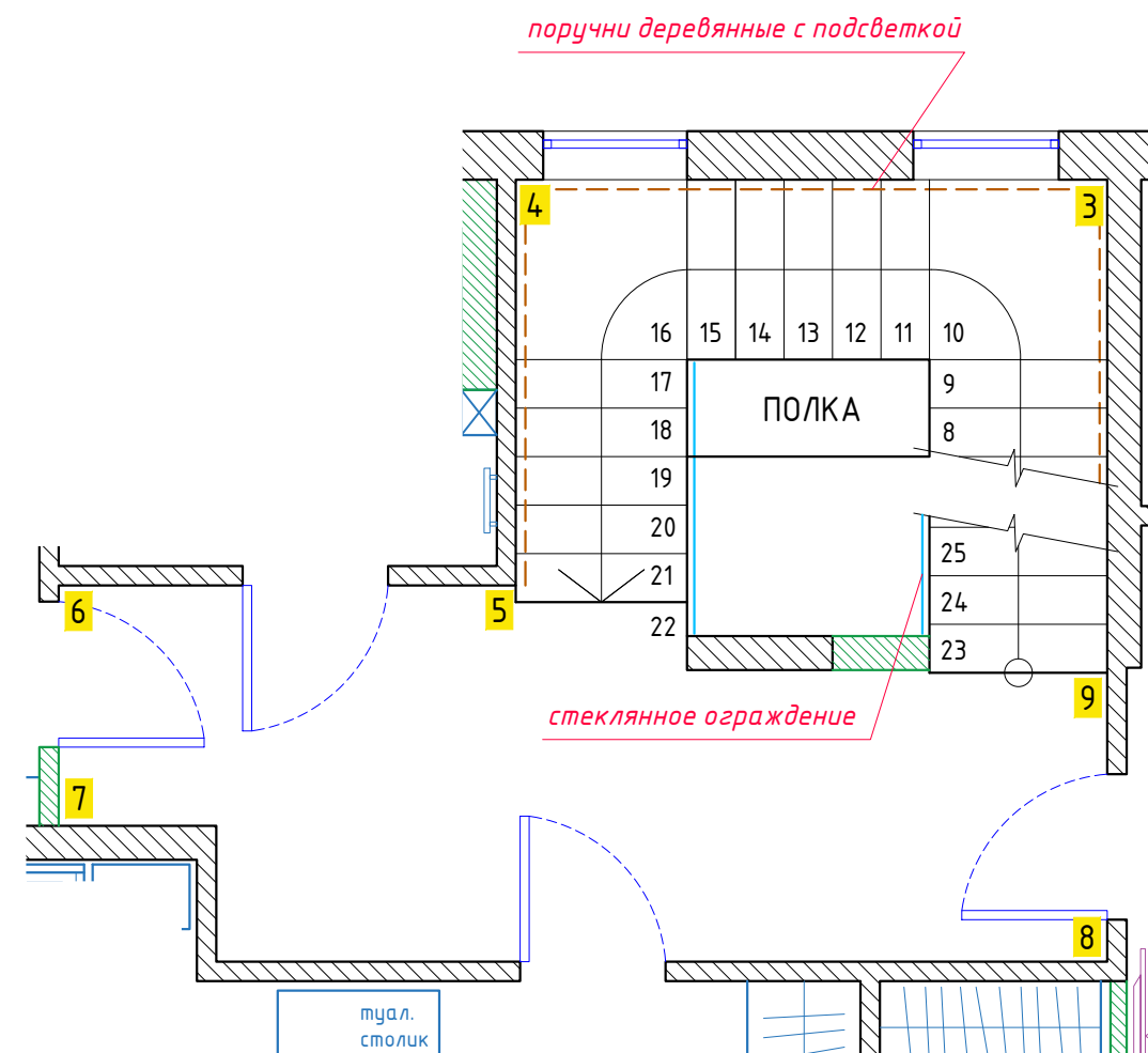
2 этаж
