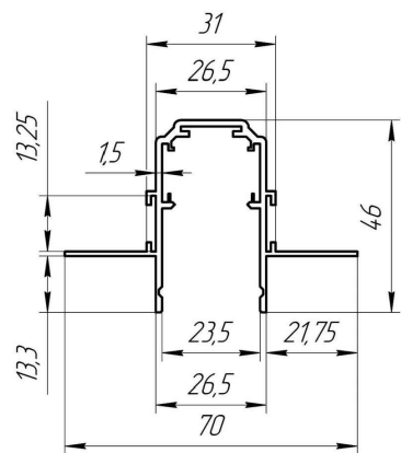
Размеры встраиваемого шинопровода под ГКЛ 12,5 мм
